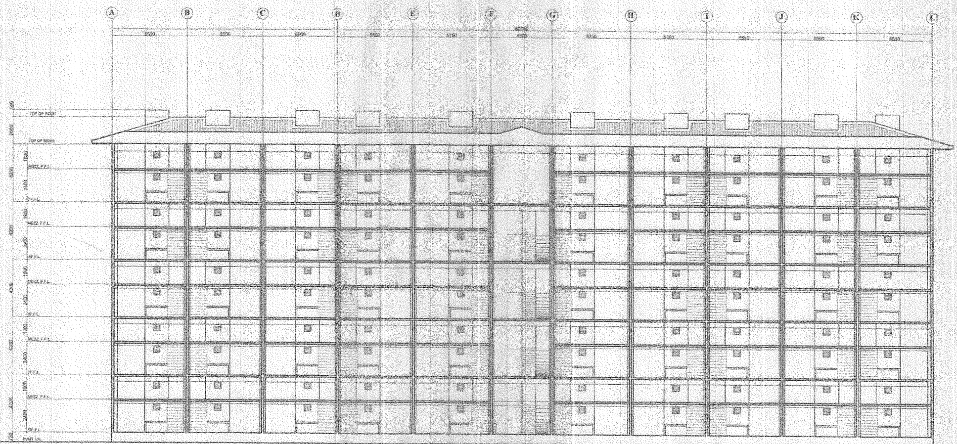
LONGITUDINAL SECTION (L) SCALE: 1:100 METS.
